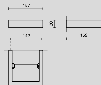
Toilettenpapierhalter / toilet roll holder Nr. 40 386E für/for USA/UK Export
