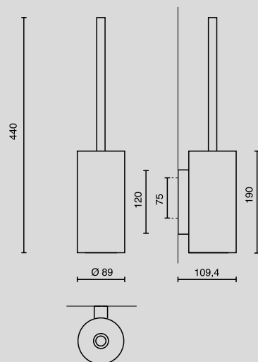
Toilettenbürste / toilet brush Nr. 40 381
