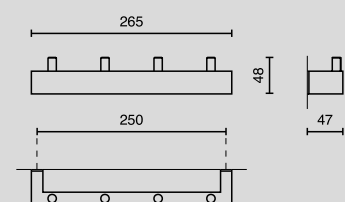
Handtuchhakenleiste / towel hook rail NR. 40 389
