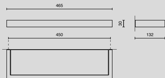
Badablage / bathroom shelf Nr. 40 384
