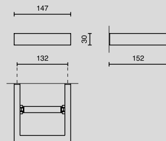
Toilettenpapierhalter / toilet roll holder Nr. 40 386
