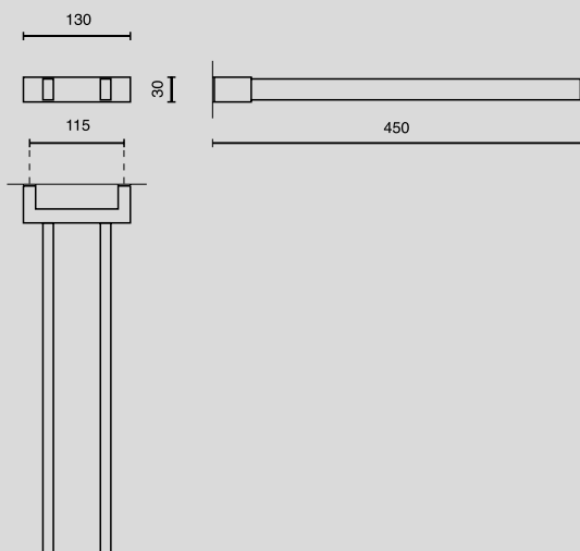
Handtuchhalter / towel holder NR. 40 392
