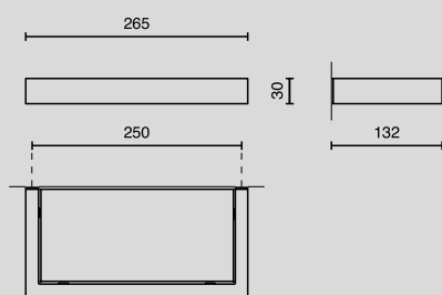
Badablage / bathroom shelf Nr. 40 383
