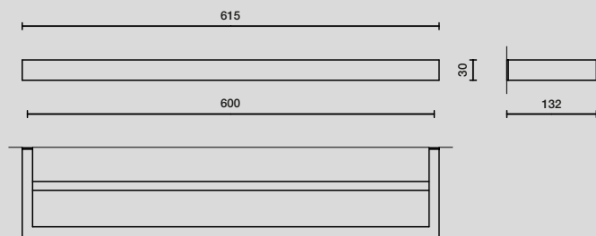
Doppel-Handtuchstange / double towel rail Nr. 40 393
