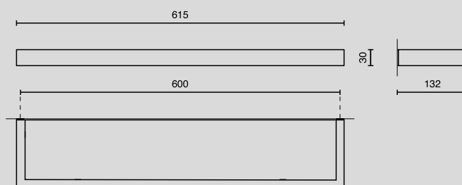
Badablage / bathroom shelf Nr. 40 385
