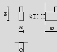
Handtuchhaken / towel hook NR. 40 395
